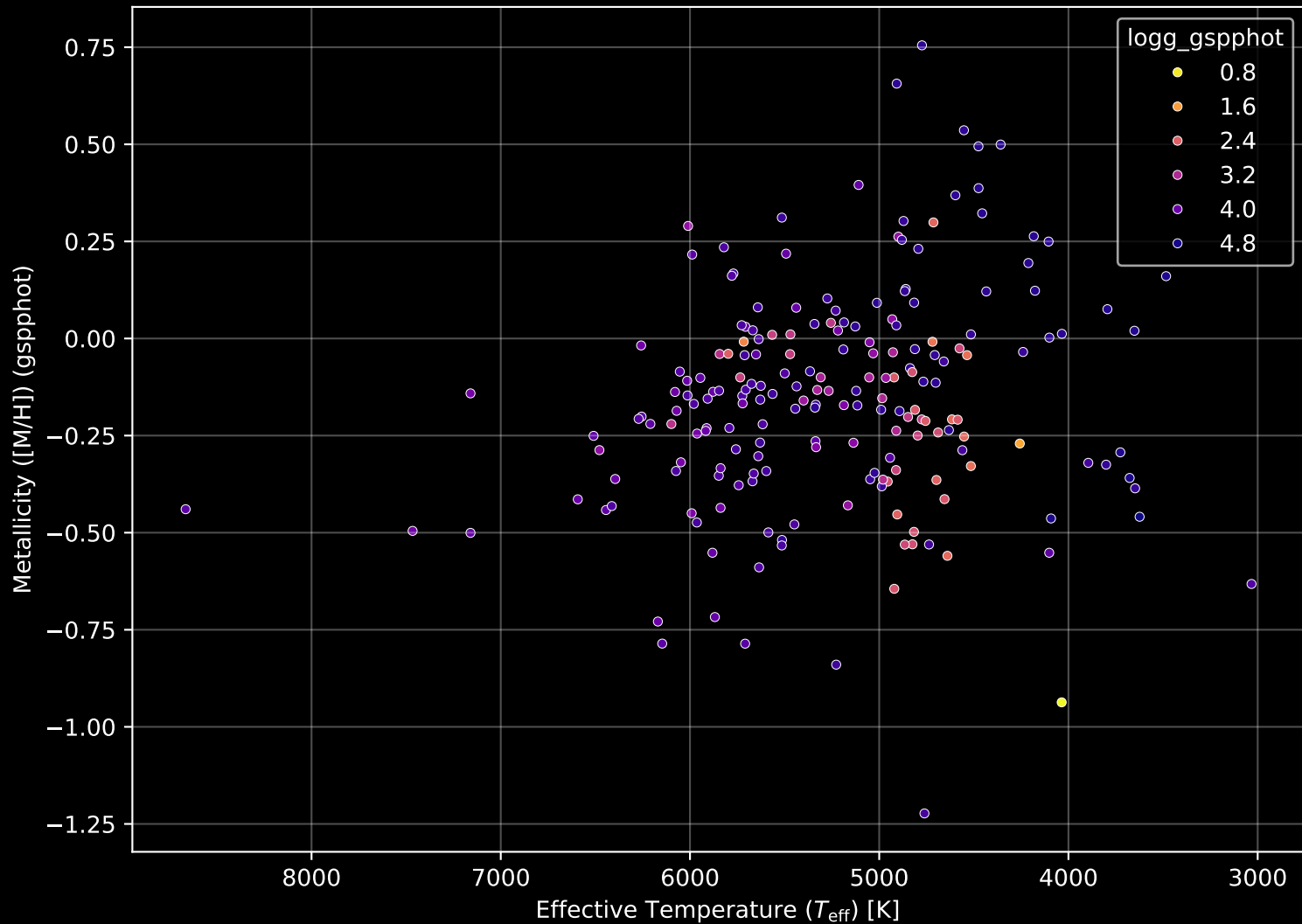
APOGEE DR17 Field: [272-38-O_TESS] Stellar Population Parameters (n= 201)
